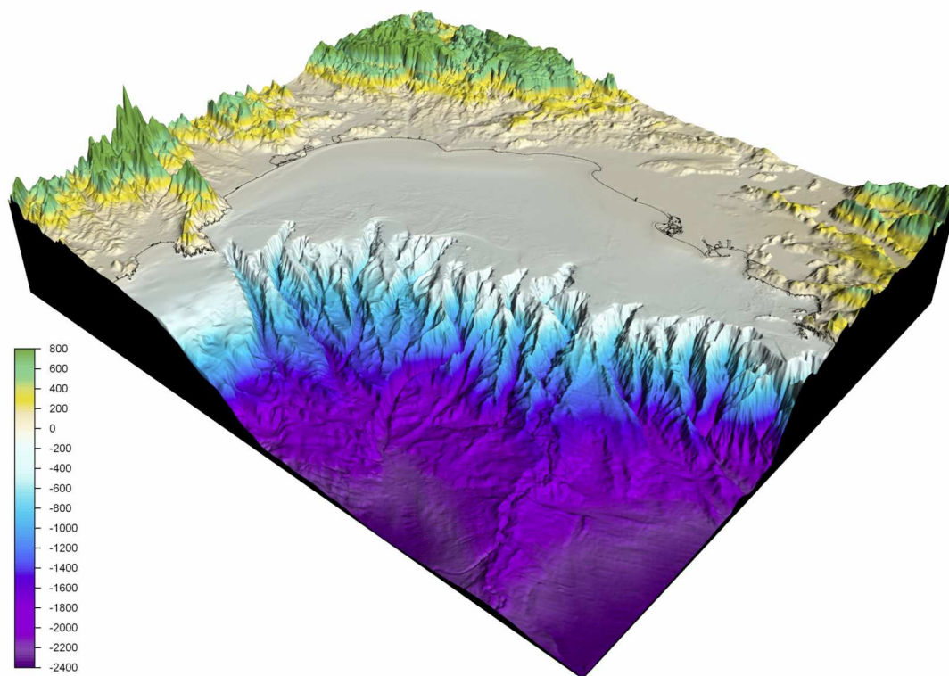
Sistema de cañones submarinos del Golfo de León, el cañón más occidental cuya cabecera se encuentra tocando el Cap de Creus es el cañón objeto de nuestro estudio. (Fuente: Serge Berné, IFREMER).
